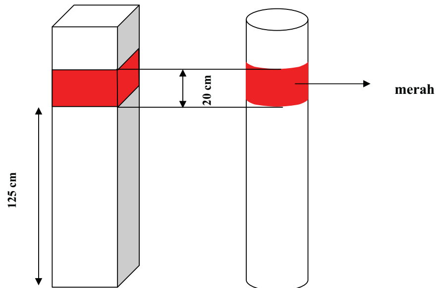
TIANG KOLOM
